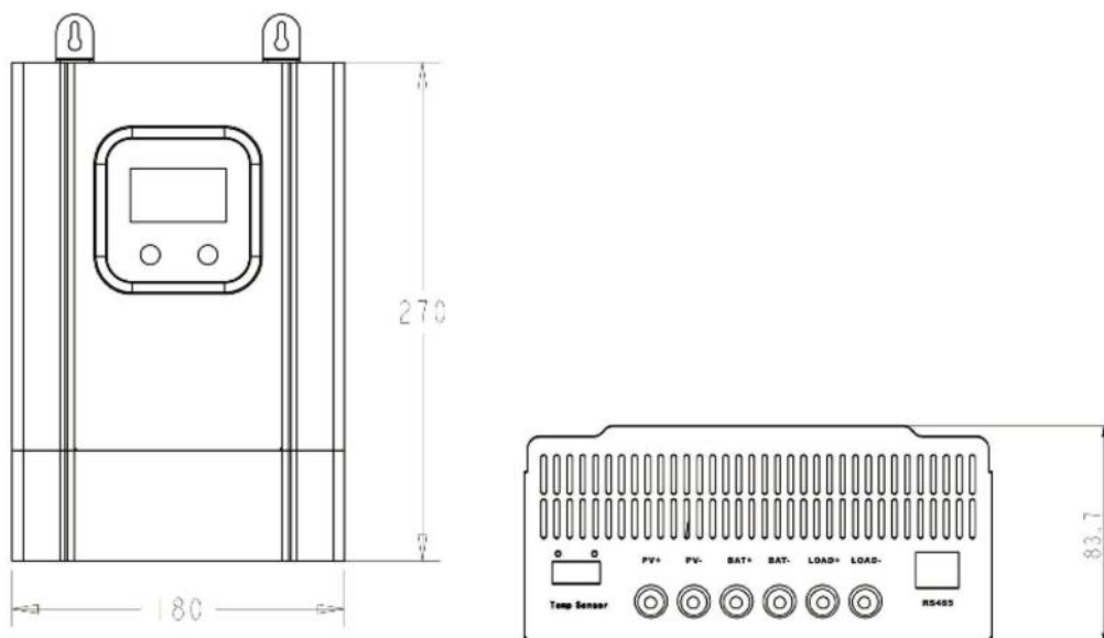
Rys. Widok regulatora: wymiary w mm. Masa 2600g
