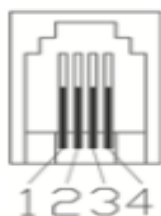
Rys 4. Położenie pinów w terminalu RJ11
