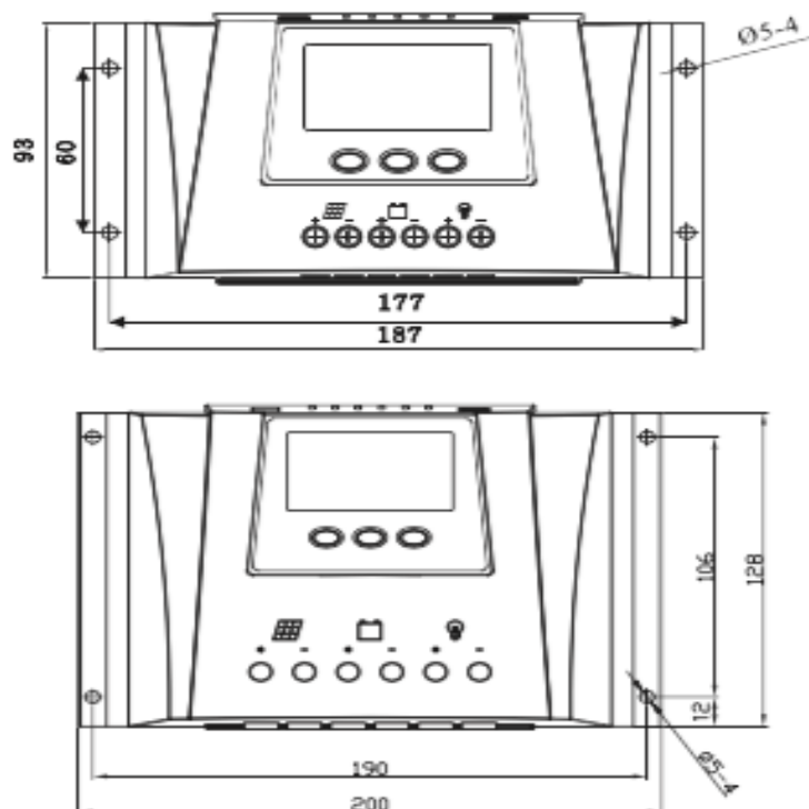
Rys 2. Rozstawy otworów montażowych w zależności od modelu
