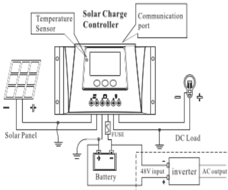
Rys 3. Schemat elektryczny dla systemu 48V. Dodatkowo pokazano podłączenie zewnętrznego inwertera wytwarzającego napięcie przemiennie AC
