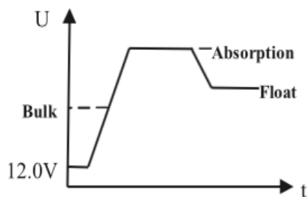
Rys 1. Tryby ładowania
