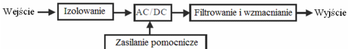
Rys.1 Schemat blokowy przetwornika jednofazowego
