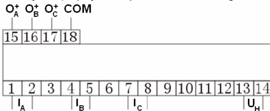
Rys. 4 Schemat podłączeń
