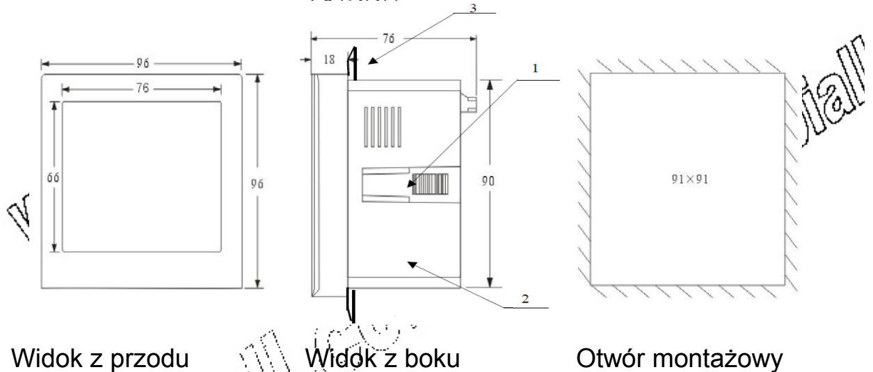
Rys. Instalacja miernika tablicowego
