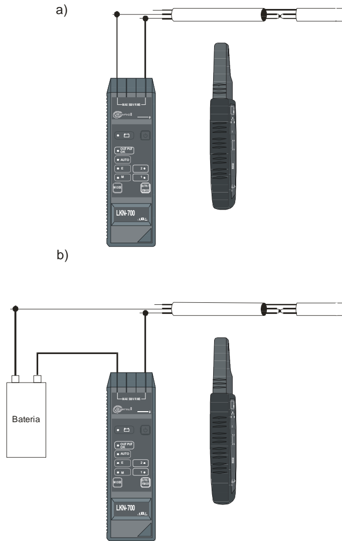
Rys.11 Lokalizacja zwarcia przewodów
