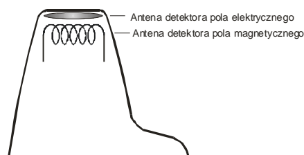
Rys.3 Umieszczenie anten detektorów w głowicy odbiornika
