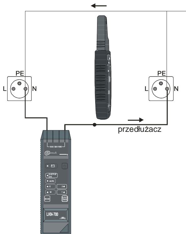
Rys.9 Lokalizowanie przewodów z zastosowaniem trybu „M+E” lub „mowego” „E”
