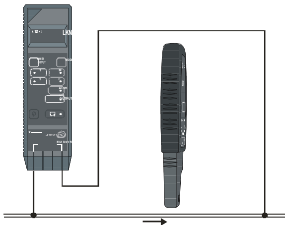
Rys.28 Śledzenie trasy rur nieziemionych z zastosowaniem trybu „M+E”
