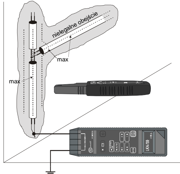
Rys.12 Wykrywanie nielegalnych obejść liczników energii elektrycznej – obejście w płaszczyźnie ściany
