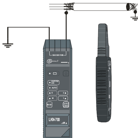
Rys.25 Śledzenie trasy kabli ekranowanych: a) tryb prądowy „M”, b) tryb prądowo-napięciowy „M+E”
