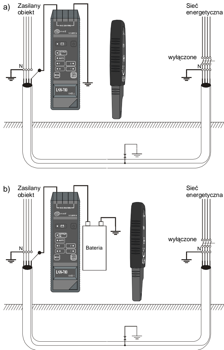
Rys.24 Lokalizowanie zwarcć doziemnych w kablach podziemnych
