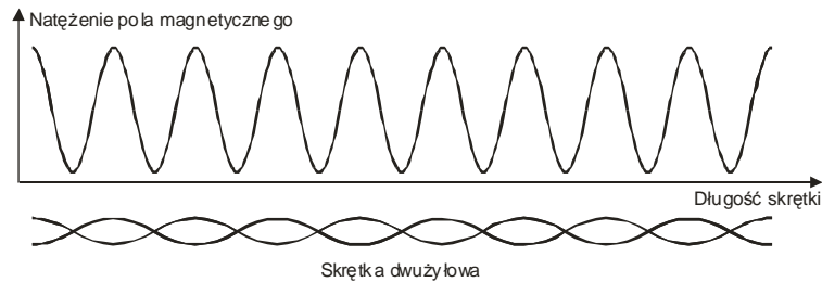
Rys.5 Rozkład natężenia pola magnetycznego wokół skrętki dwużyłowej
